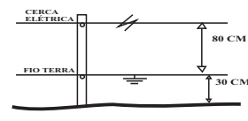
DISPOSIÇÃO DOS FIOS NA CERCA ELÉTRICA, CONSIDERANDO A ESPÉCIE ANIMAL E A CONDUTIVIDADE DO SOLO
